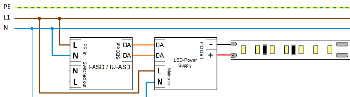
Typisches Schaltbild Typical connection scheme
